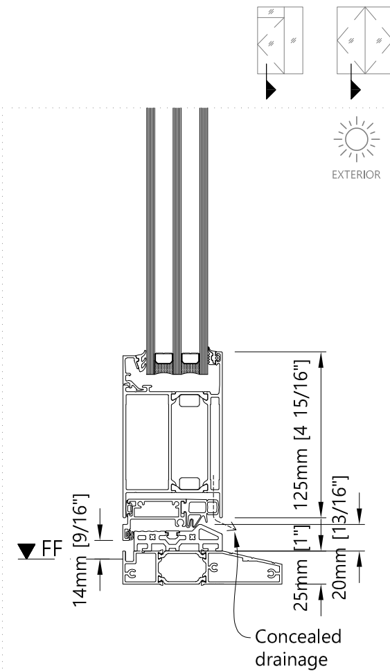
Bottom - Vertical Single/Double Inswing door
