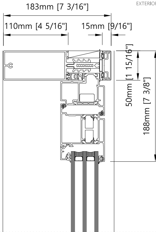
Top - Vertical Single/Double Inswing door
