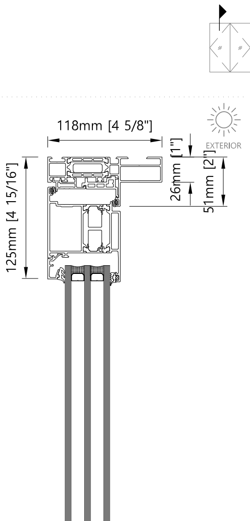
Top - Vertical Single/Double Inswing door
