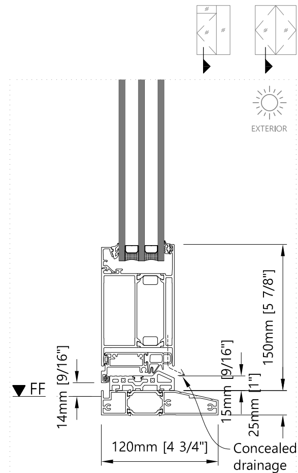
6 Bottom - Vertical Single/Double Inswing door
