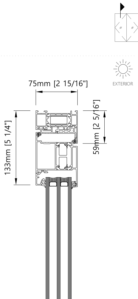
4 Top - Vertical Single/Double Inswing door
