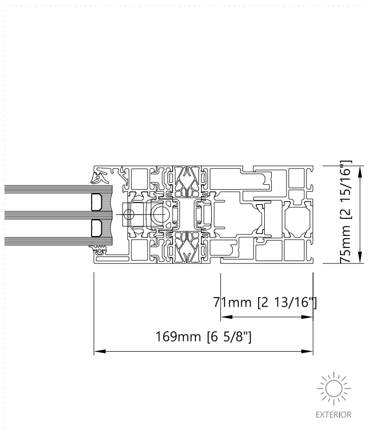
Jamb - Horizontal Inswing bi-folding door
