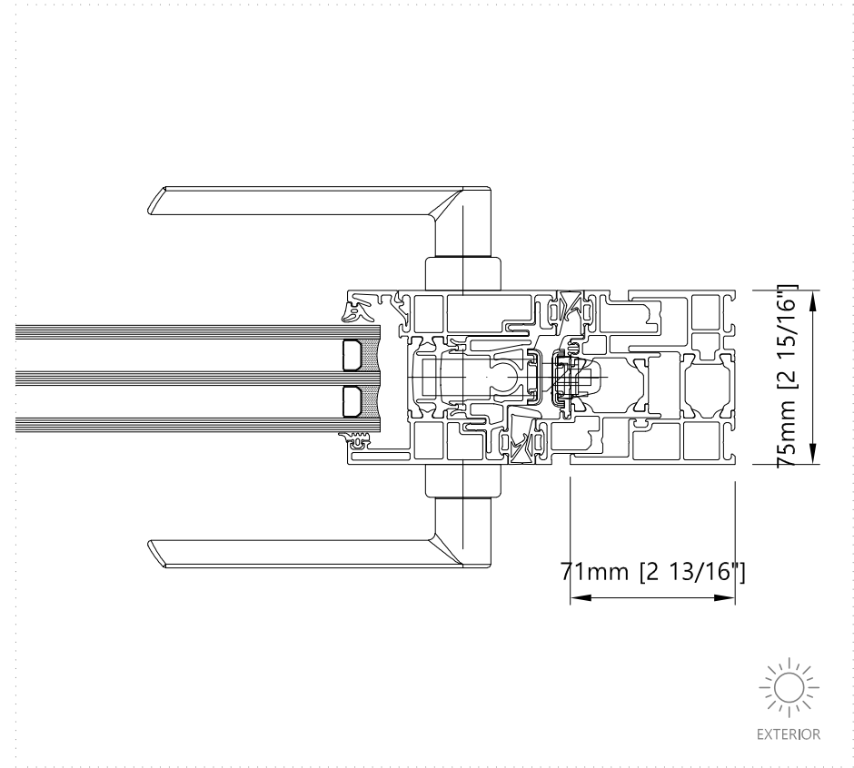
4 Jamb - Horizontal Inswing bi-folding door
