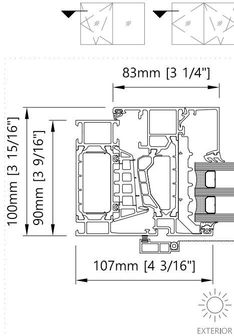
5 Jamb - Horizontal T&T Window / Double T&T
