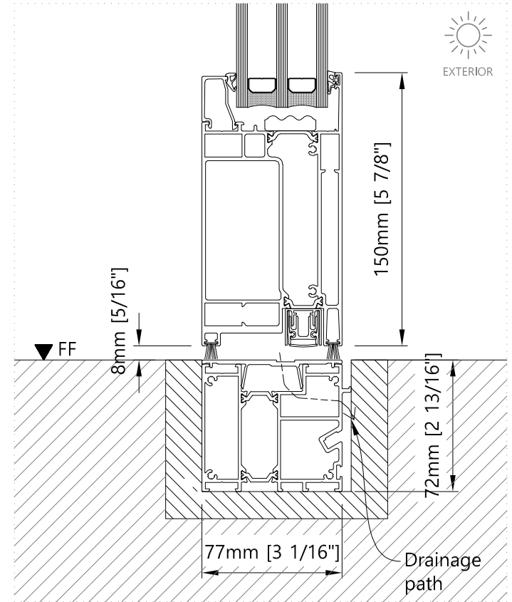
Bottom - Vertical Pivot XL Inswing door
