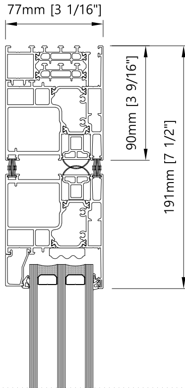
Top - Vertical Pivot XL Inswing door
