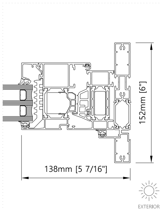
Jamb - Horizontal Single terrace door
