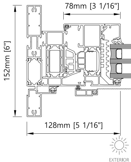
Jamb - Horizontal T&T Window / Double T&T
