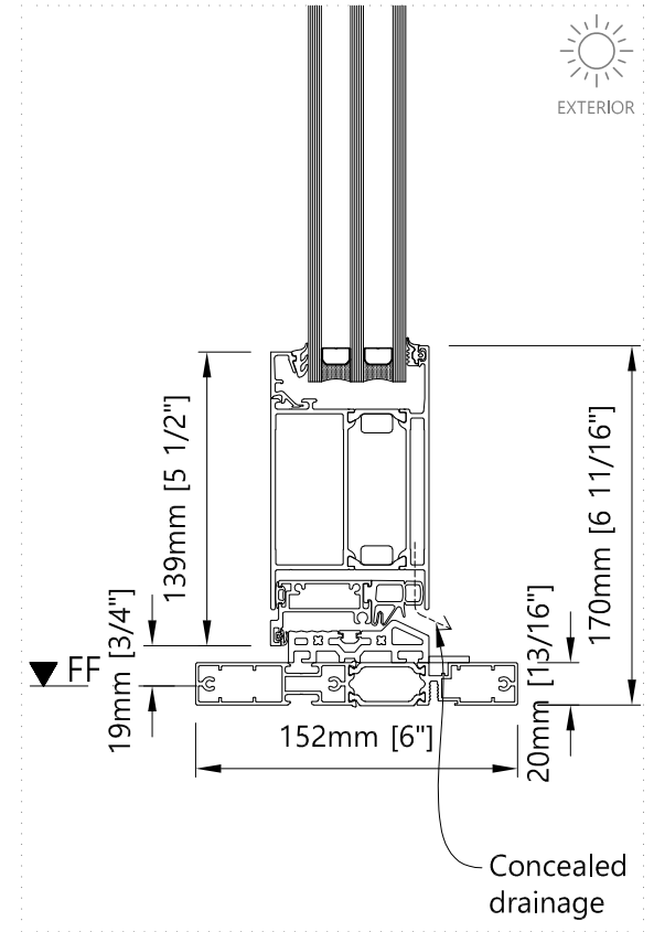
Bottom - Vertical Single/Double Inswing door
