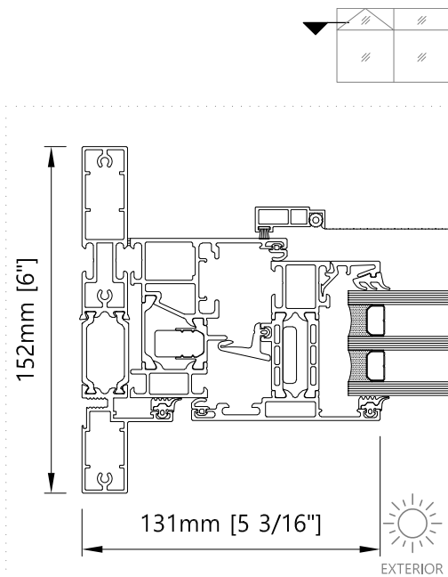
Jamb - Horizontal Motorized awning
