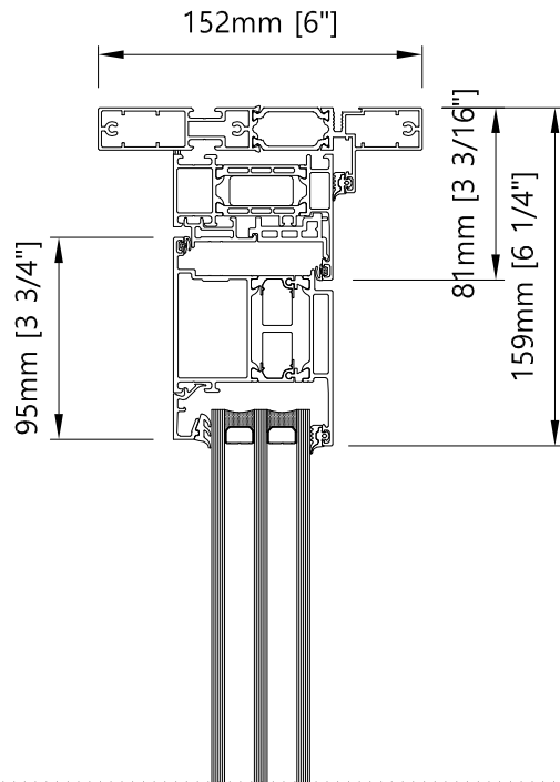
Top - Vertical Single/Double Inswing door
