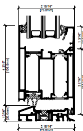
AD UP 75 BL Sill
