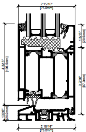
AD UP 75 Sill
