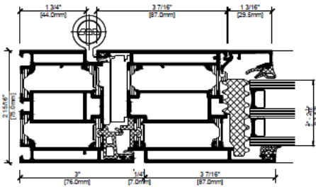
AD UP 75 Jamb
