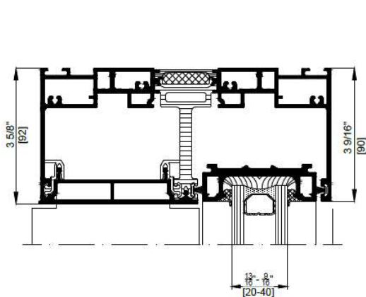
ASS 77 PD.HI Head
