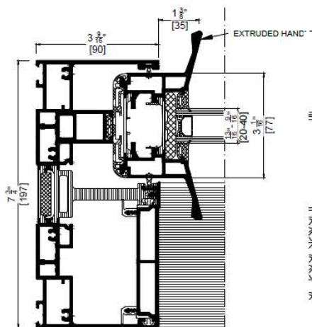
ASS 77 PD.HI Jamb
