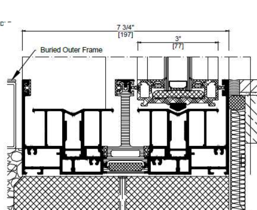
ASS 77 PD.HI Sill
