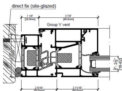
AWS 70.Hi jamb
