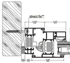
AWS 70.HI jamb
