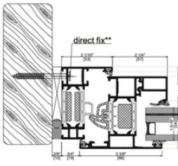
AWS 75.SI jamb
